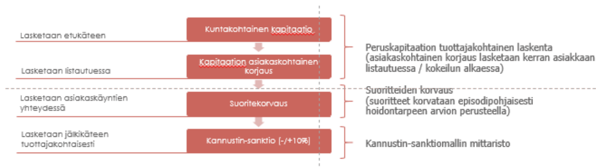
Kuva 5 Korvausten laskentaperiaatteet
