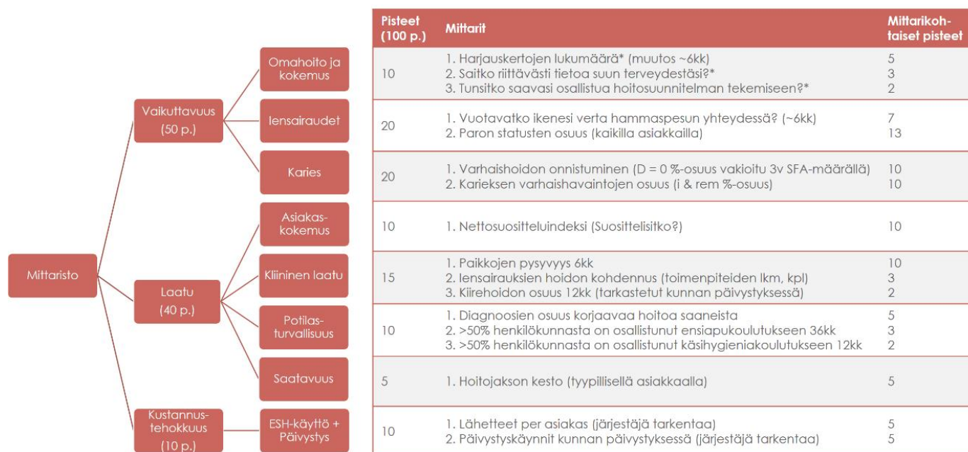
Kuva 10 Kannustin-/sanktiojärjestelmän mittaristo
